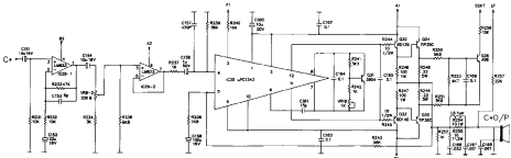
Schallbild Verstärker Teil 3 - Circuit diagram amplifier Part 3
